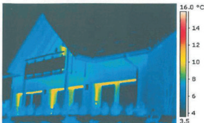
Photo caméra thermique
